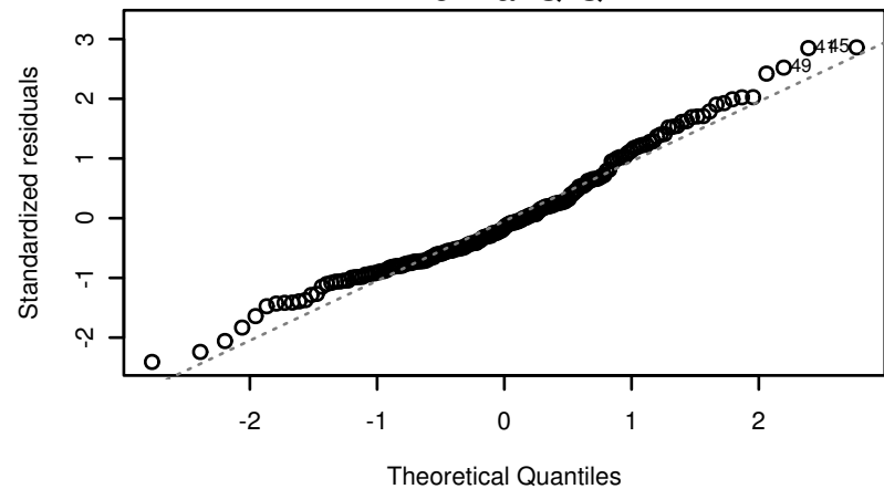
Normal Q-Q
