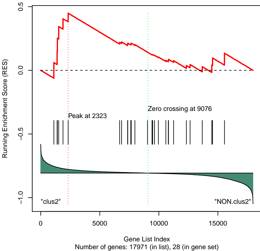
Gene Set 44 : BIOCARTA_VEGF_PATHWAY
