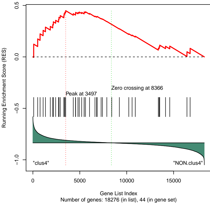
Gene Set 13 : KEGG_VALINE_LEUCINE_AND_ISOLEUCINE_DEGRADA
