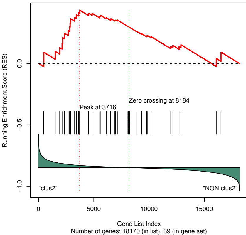
Gene Set 307 : PID_ECADHERIN_NASCENTAJ_PATHWAY
