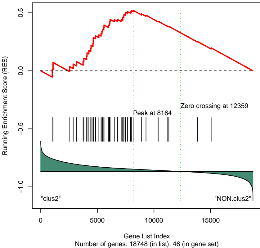
Gene Set 230 : PID_FANCONI_PATHWAY
