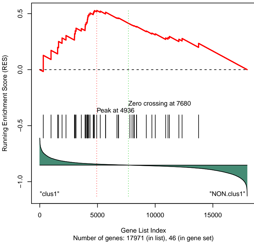
Gene Set 294 : PID_TNFPATHWAY
