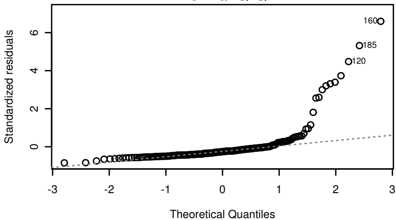
Normal Q-Q
