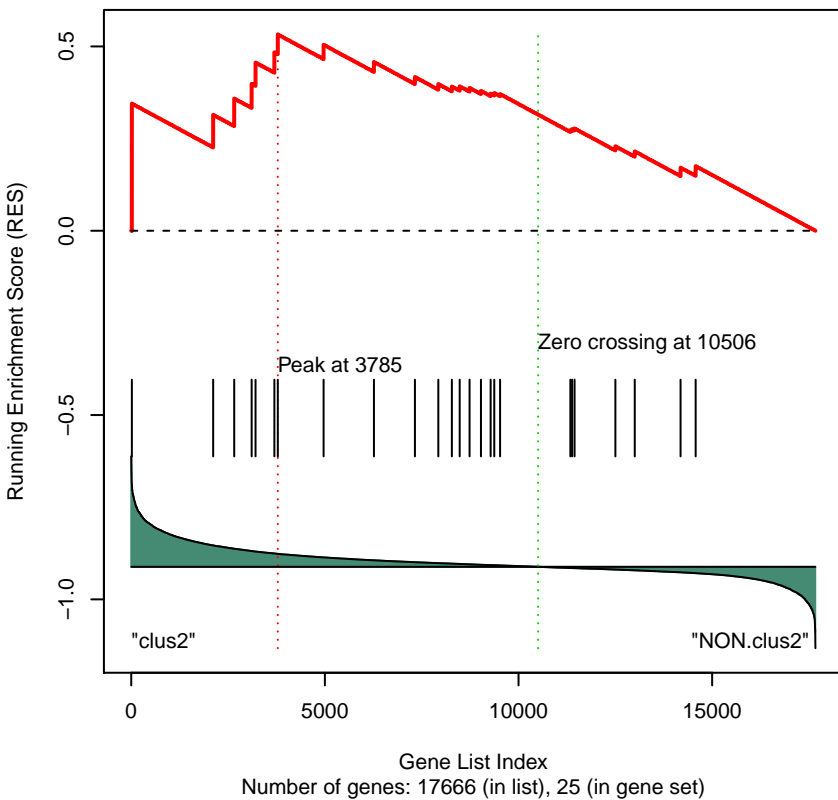
Gene Set 175 : BIOCARTA_VIP_PATHWAY
