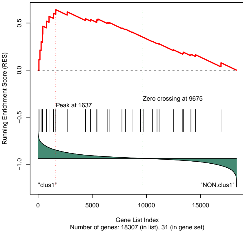
Gene Set 352 : PID_AURORA_A_PATHWAY
