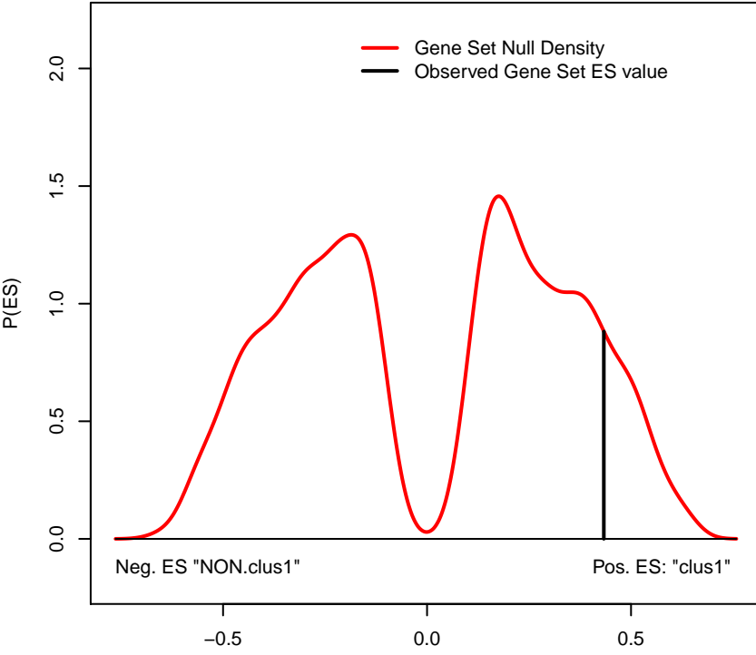
ES ES = 0.433 NES = 1.44 Nom. p-val= 0.201 FWER= 0.995 FDR = 1
