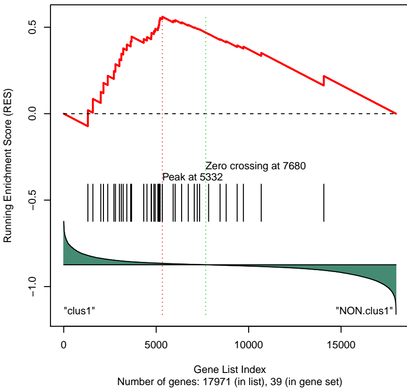
Gene Set 305 : PID_ECADHERIN_NASCENTAJ_PATHWAY
